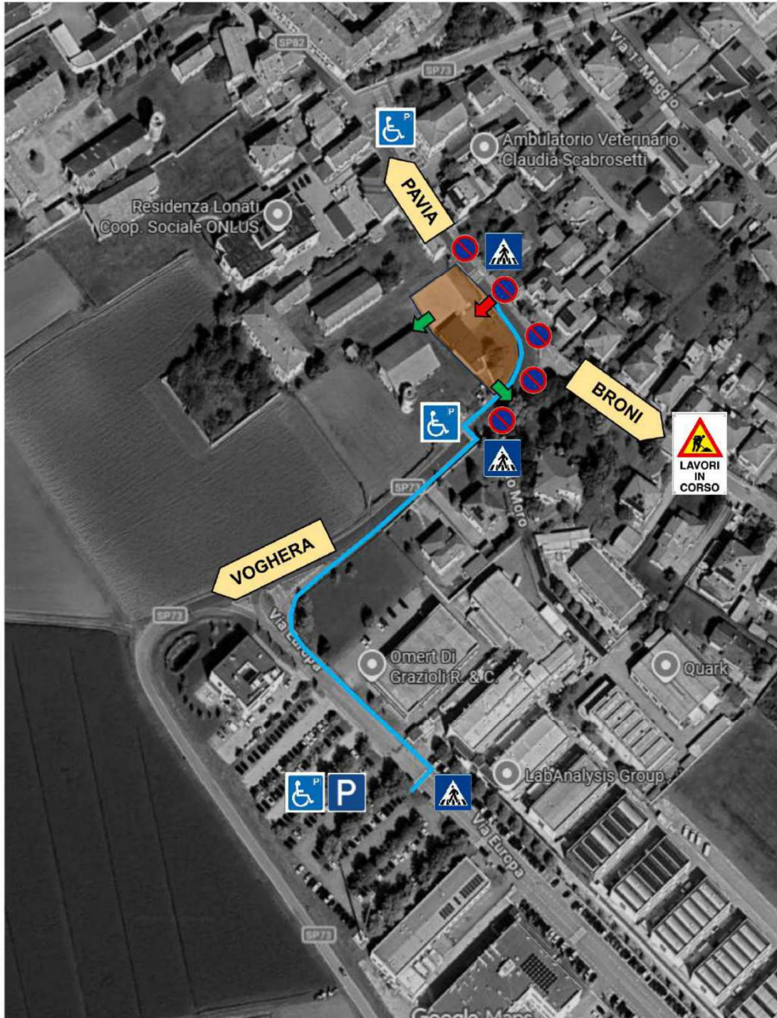
TAVOLA 2 - PLANIMETRIA VIABILITÀ ESTERNA, PARCHEGGI E PERCORSO PEDONALE
